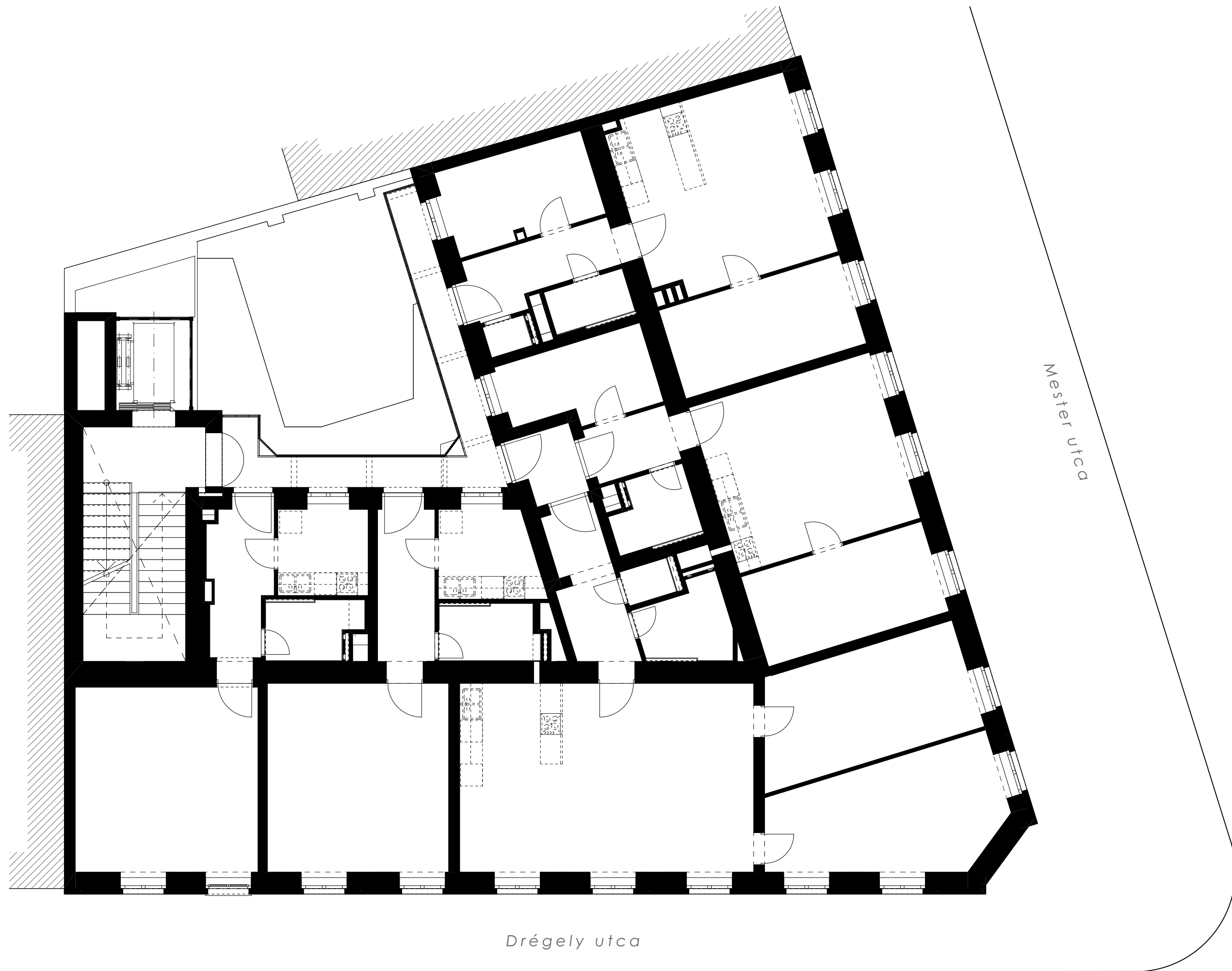
1. emeleti alaprajz
