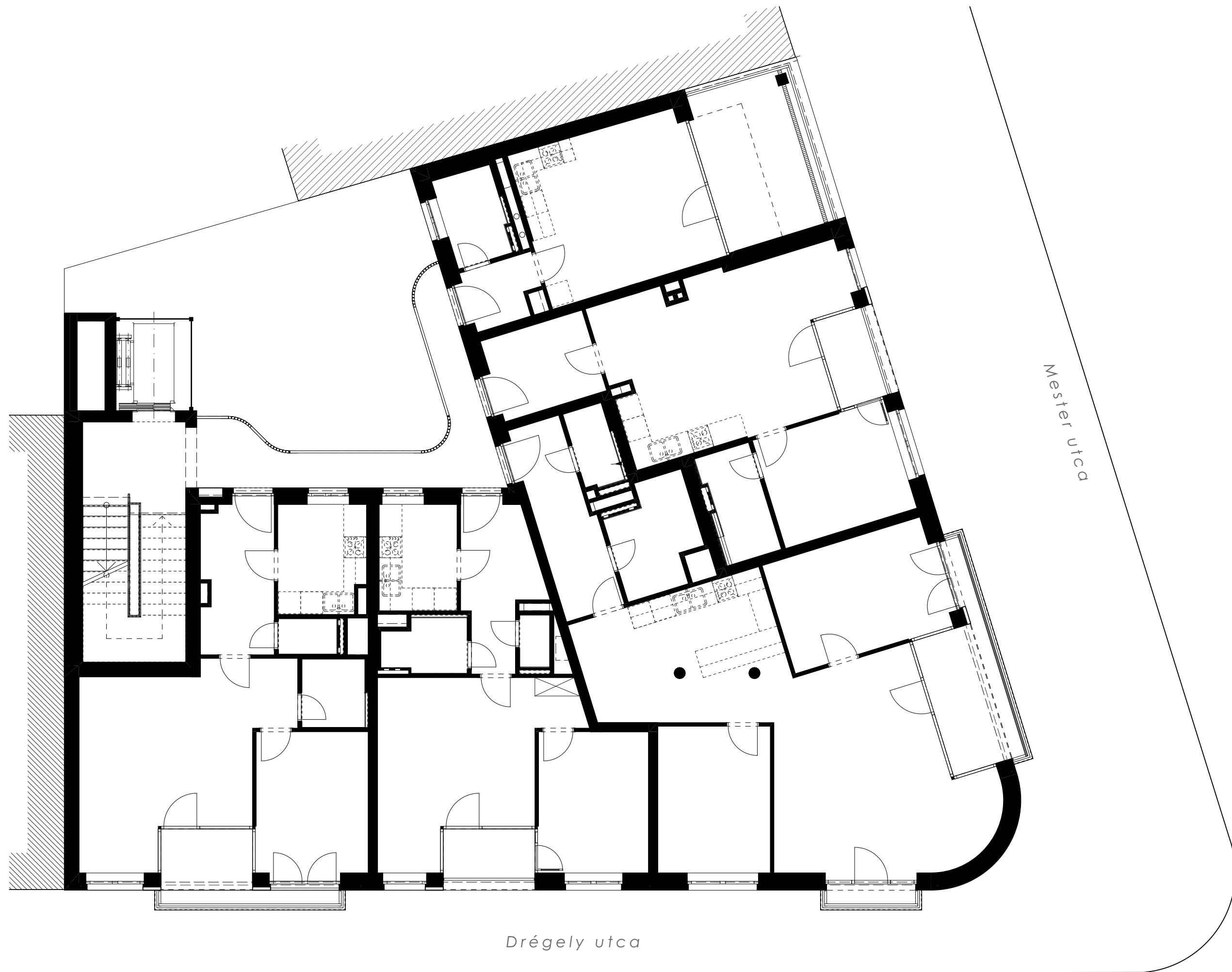
4. emeleti alaprajz
