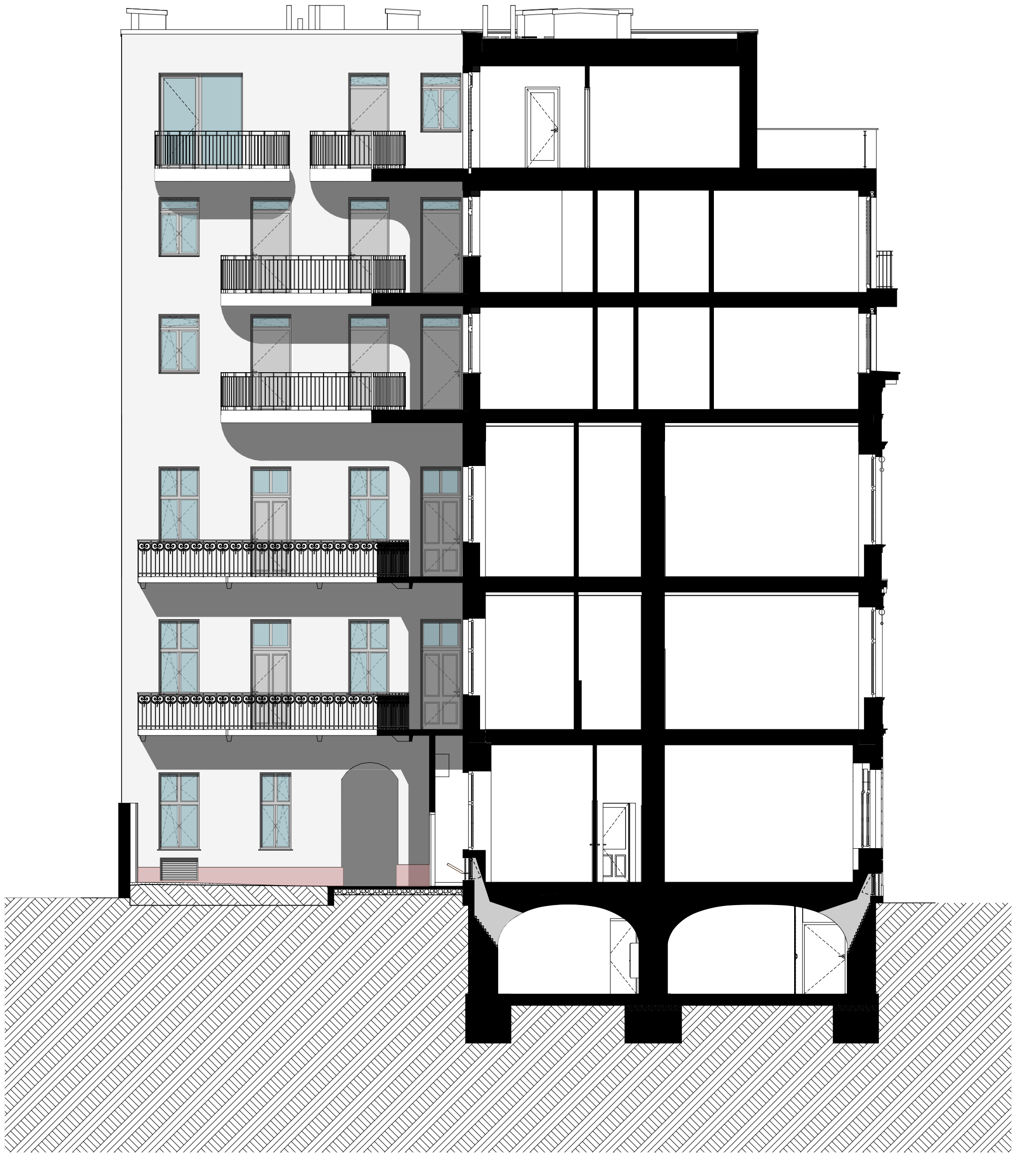
A-A metszet
