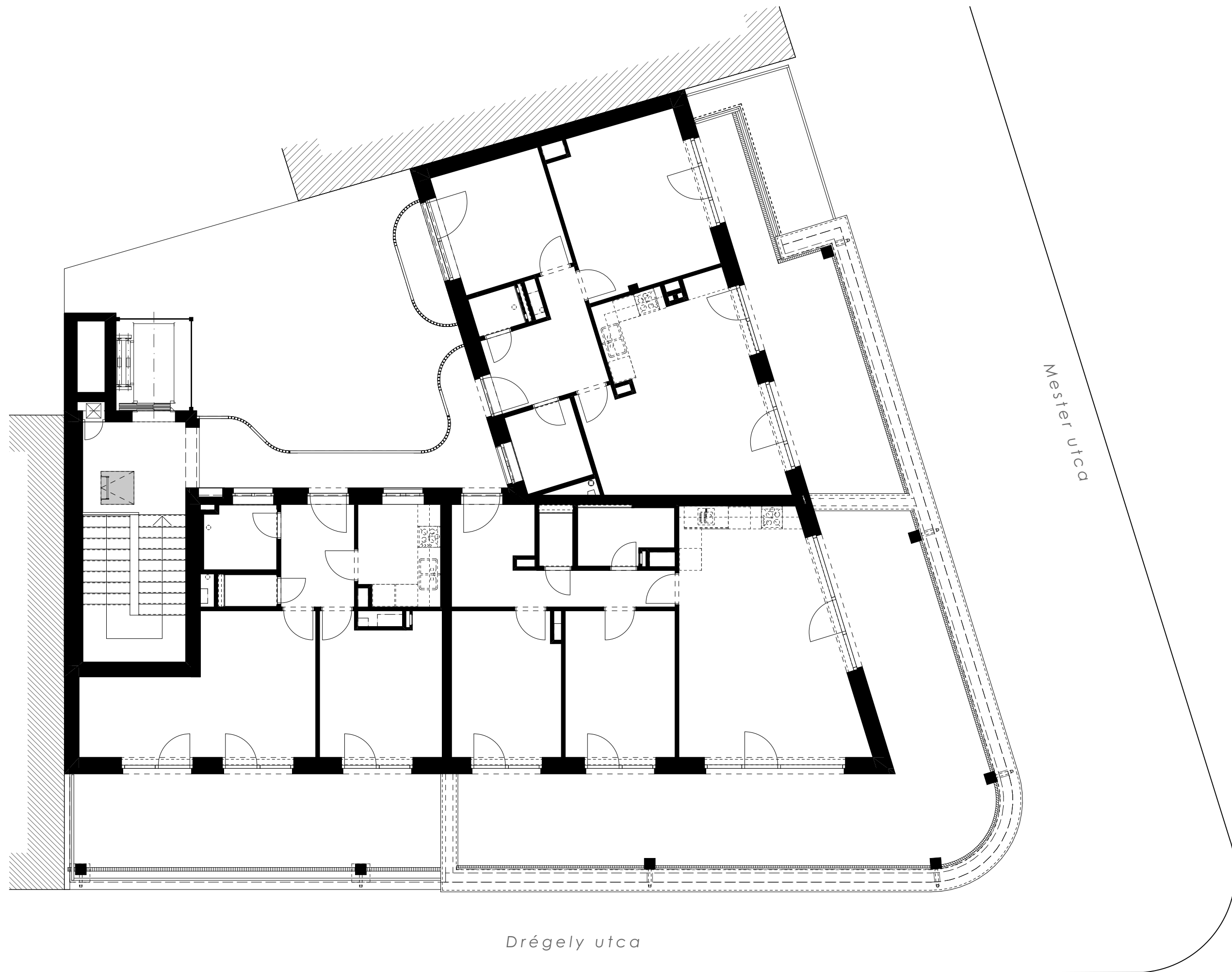
5. emeleti alaprajz
